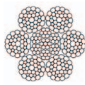
6xK36WS - PWRC
