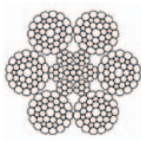
6xK36WS - IWRC
