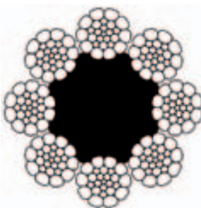
8xK26WS – FC
