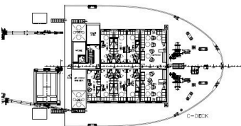
C-DECK
