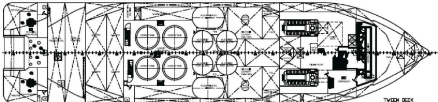
TWEEN DECK
