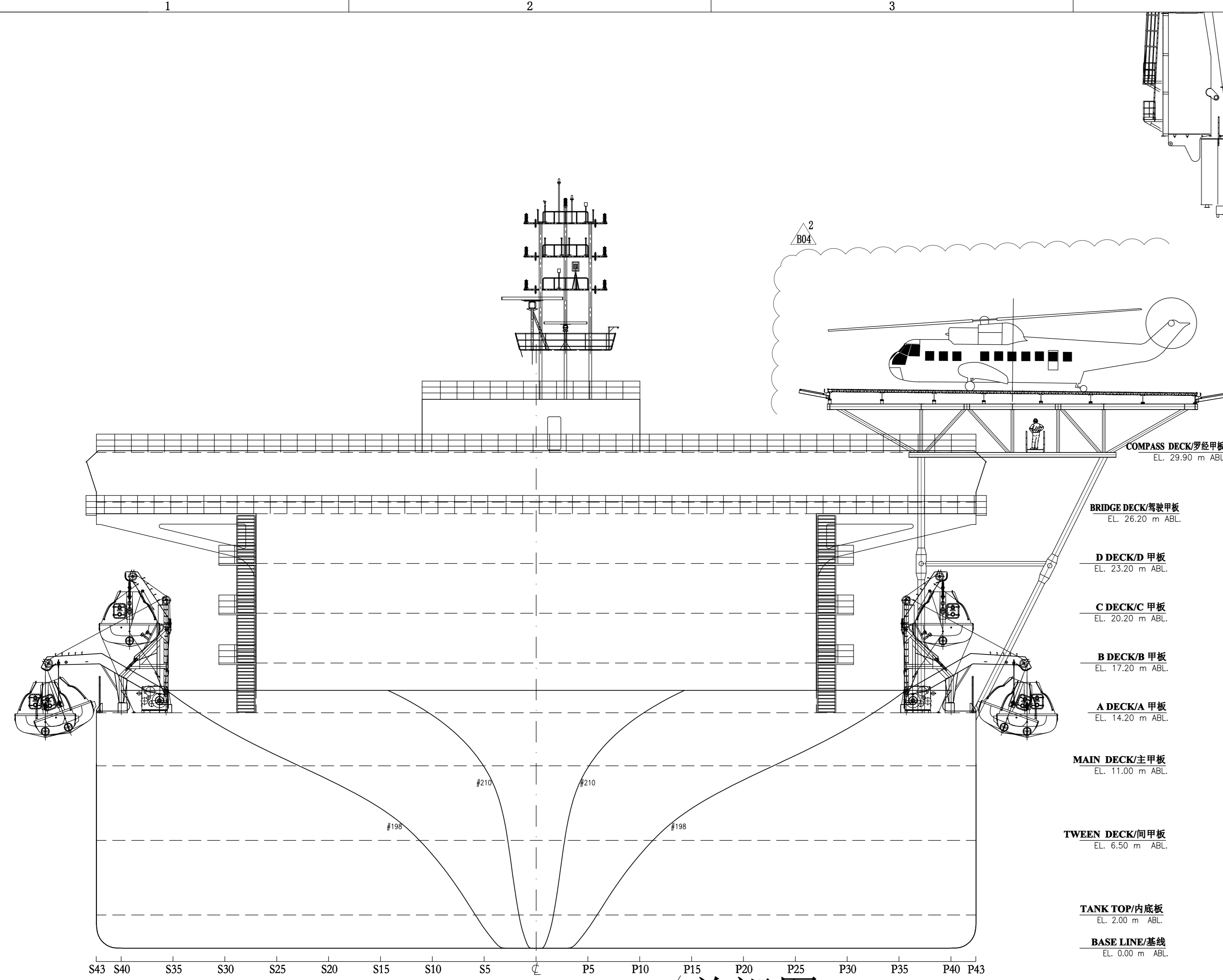
FWD VIEW / 首视图 LOOKING AFT / 向尾看
