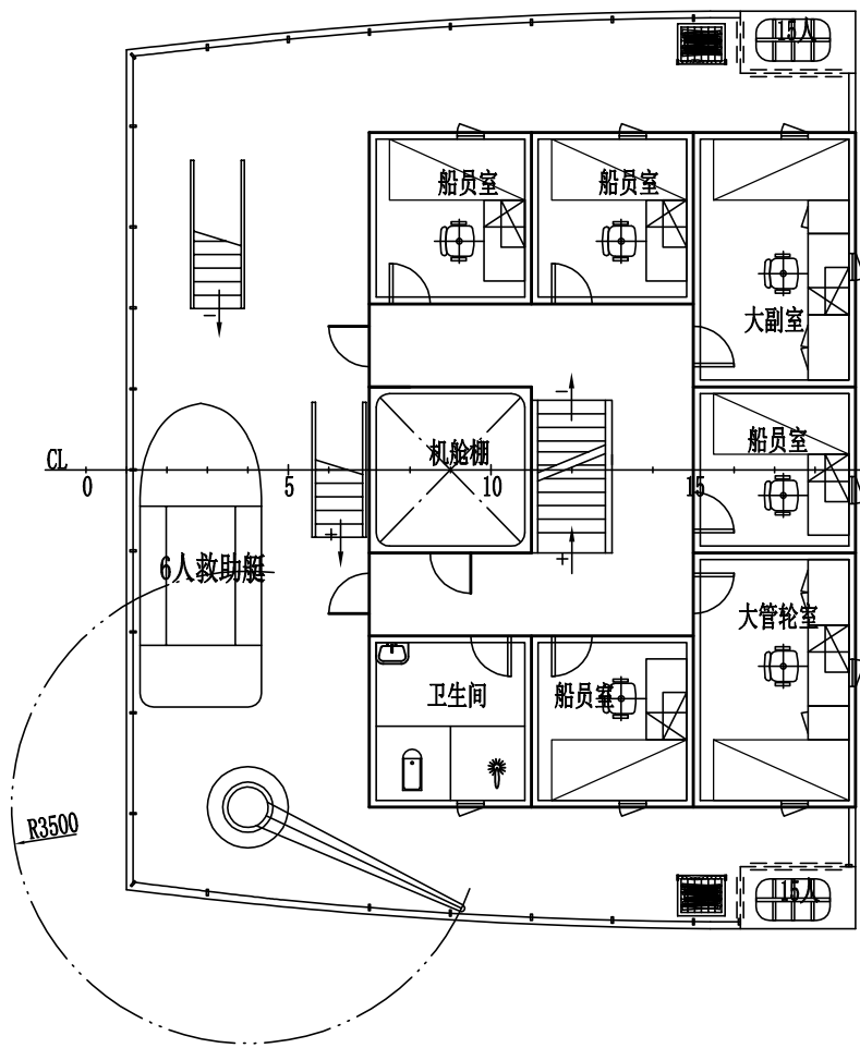
救生甲板
