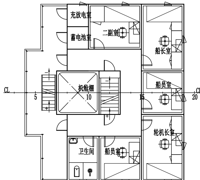
船长甲板
