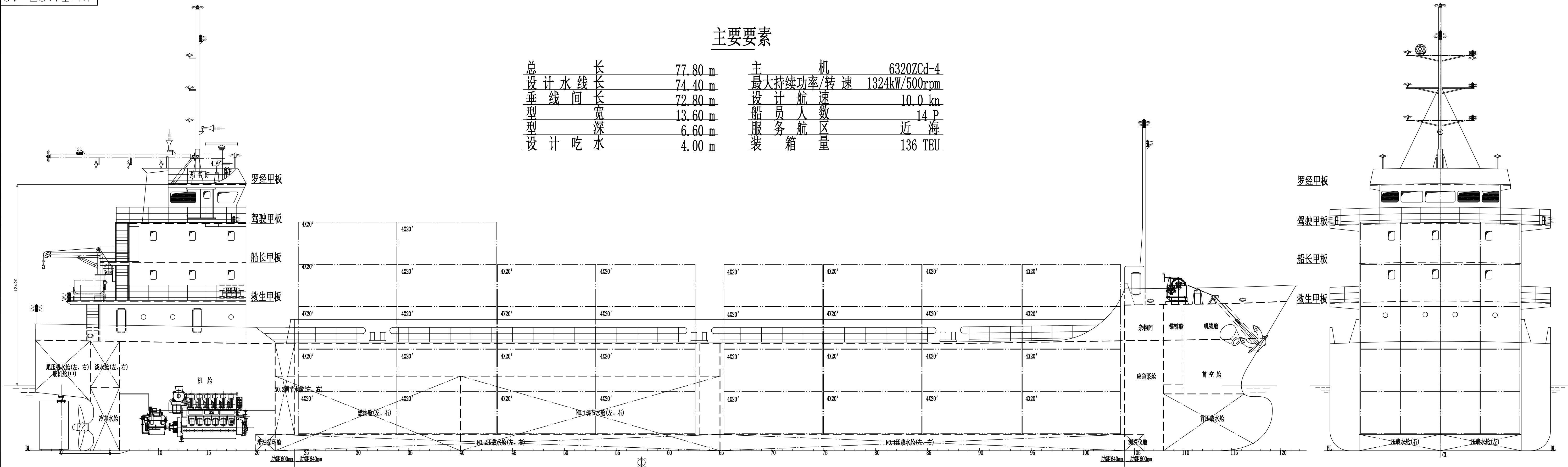
首楼甲板
