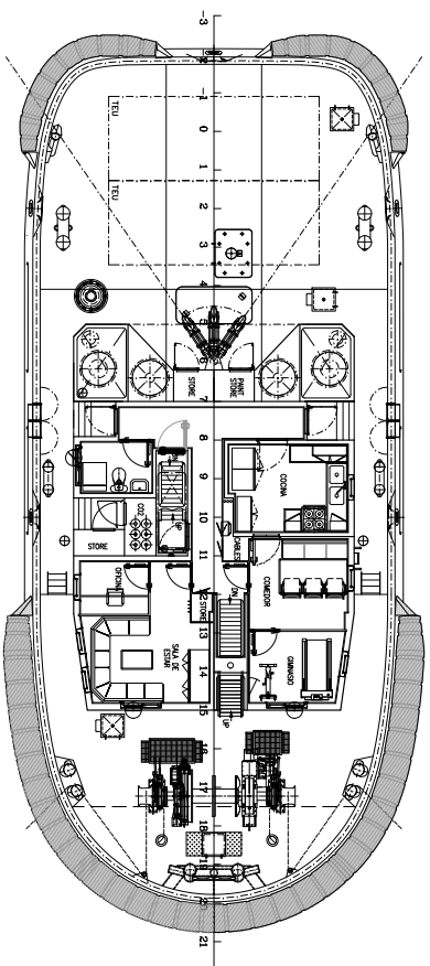
CUBIERTA PRINCIPAL
