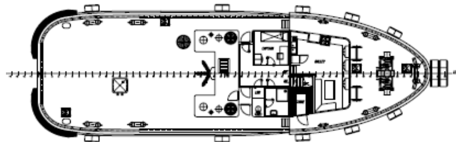
CUBIERTA PRINCIPAL
